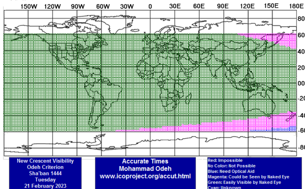
Gambar 2. Kenampakan Hilal pada Hari Selasa 21 Februari 2023 dilihat dengan mata telanjang pada garis matla' 120'
