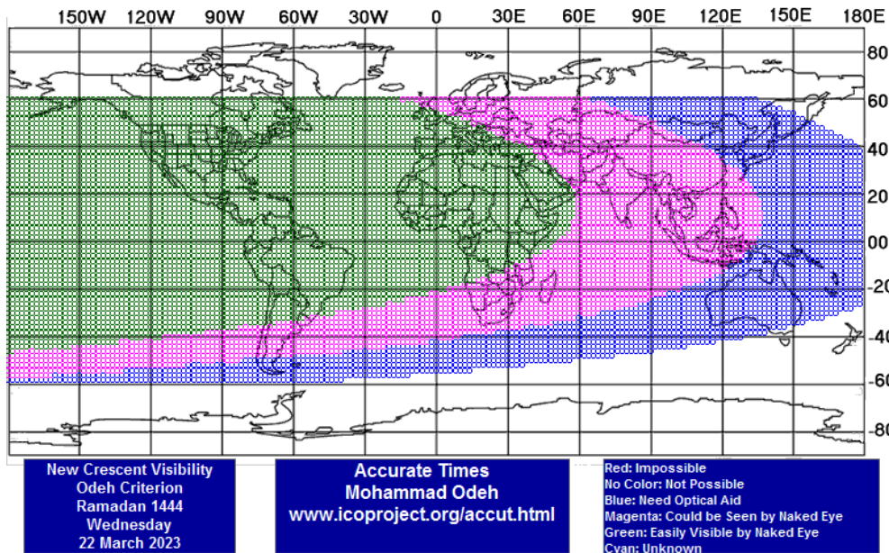
Gambar 3. Kenampakan Hilal pada Hari Rabu 22 Maret 2023 tidak terlihat dengan mata telanjang pada garis matla' 120' (Sumber: The Accurate Time)
